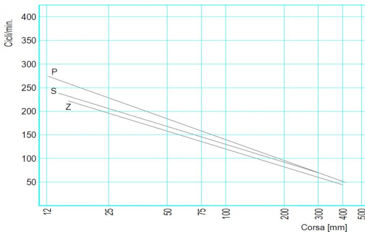
Diagramma cicli/minuto
